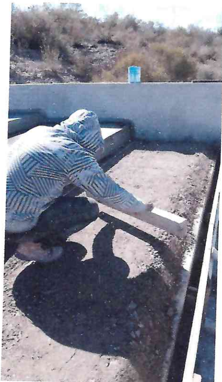
CORRECCION DE GRADAS CON PROBLEMAS DE CAIDA DE HUELLA, USO DE RELLO DE TIERRA COMPACTADA
