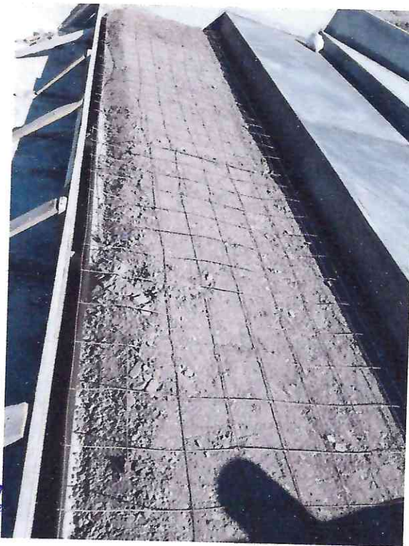
SUBDIVISION DE HUELLAS, USO DE MADERA Y REFUERZO DE MALLA ELETROSOLDADA 6- 6, APRECIZACION DE HULLAS CORREGIDAS
