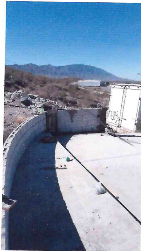
ACABADO APARENTE DE MURO LATERALES, LISTOS PARA SER SARPEADOS
