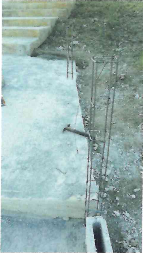
COLOCACION DE CASTILLOS A EQUIDISTANCIAS, PARA AMARRE DE BLOCK'S
